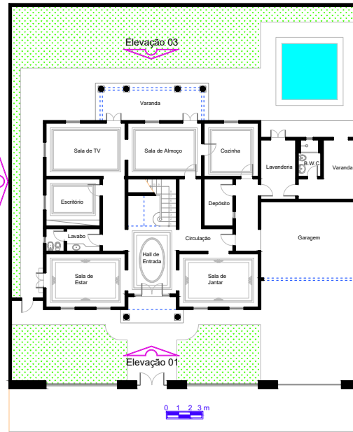
Térreo
