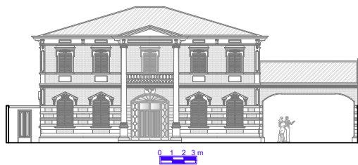
Elevação 01
