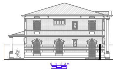
Elevação 02
