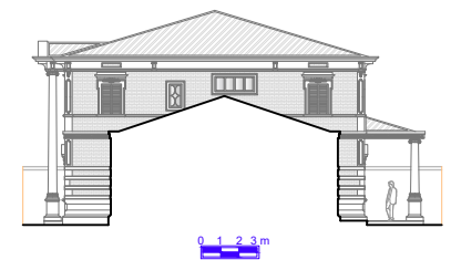
Elevação 04
