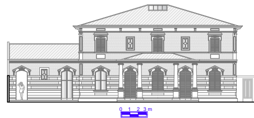
Elevação 03
